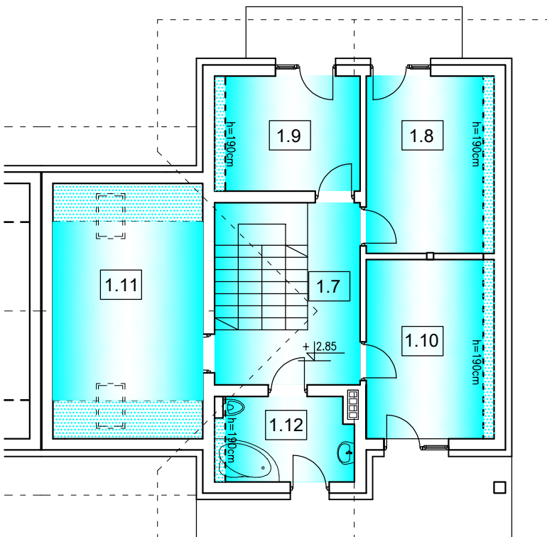
PODDASZE
